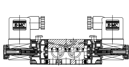
双电控电磁阀
