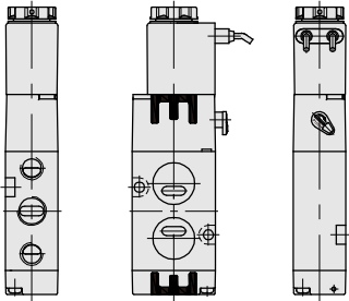
引出线式
