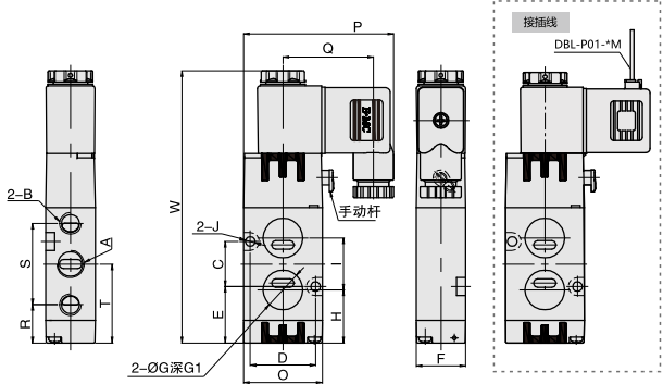
接线盒式
